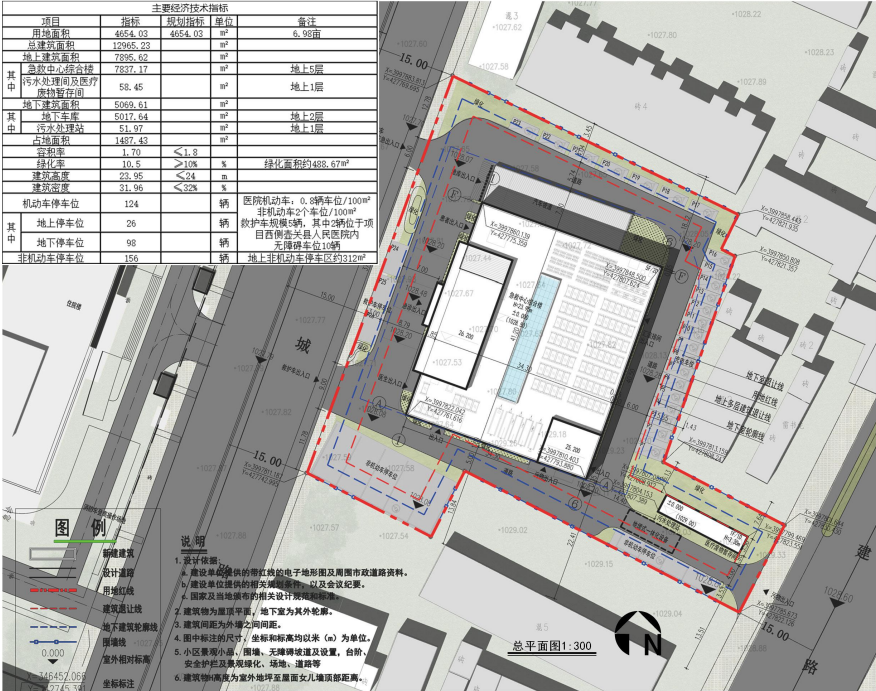
壶关县人民医院急救中心综合楼总平面图
